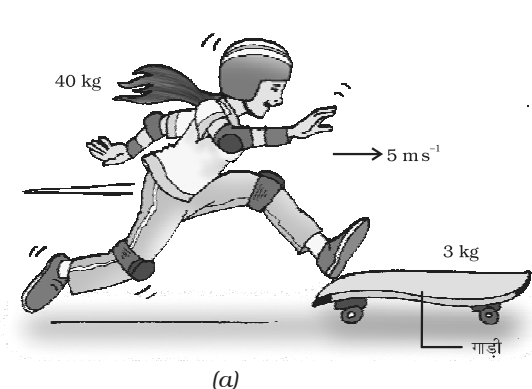
चित्र 9.18: लड़की गाड़ी पर कूदती है
