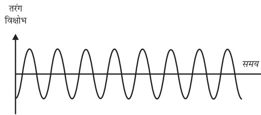
उच्च तारत्व की ध्वनि की तरंग
