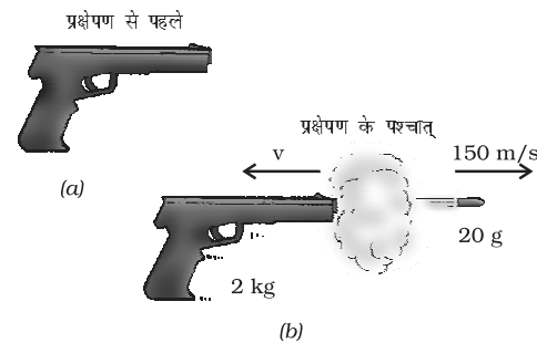
चित्र 9.17: पिस्टल का प्रतिकक्षेपण
