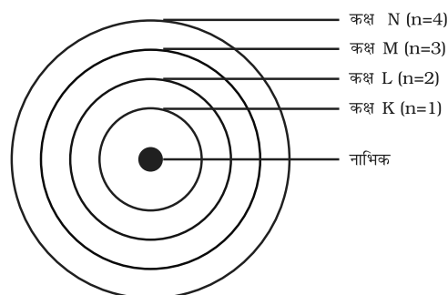
चित्र 4.3: किसी परमाणु में कुछ ऊर्जा स्तर
