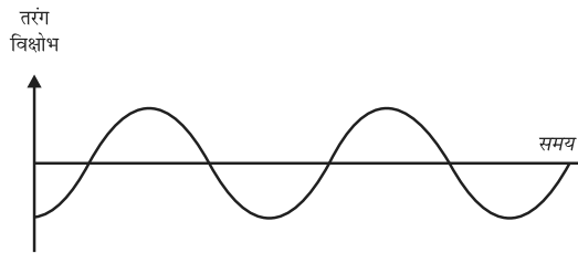
निम्न तारत्व की ध्वनि की तरंग
